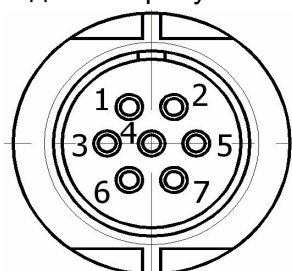
Рисунок 1. РС-7 Розетка
